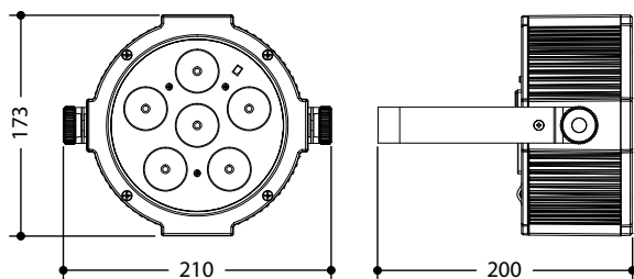
Disegno tecnico
